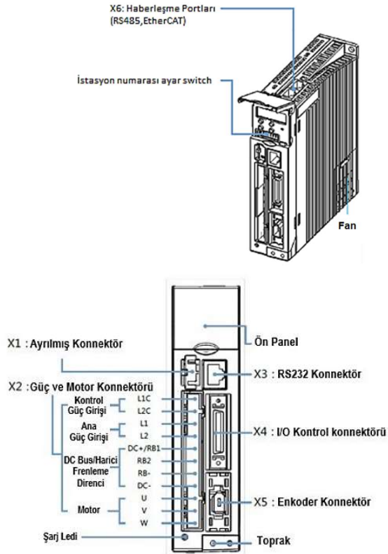
GSS3-2XX Sürücü görünümü
