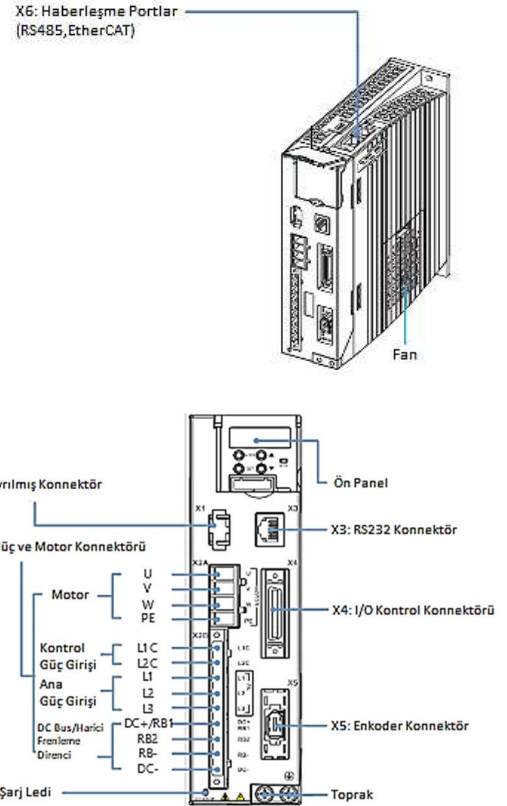
GSS3-3XX / GSS3-4XX Sürücü görünümü
