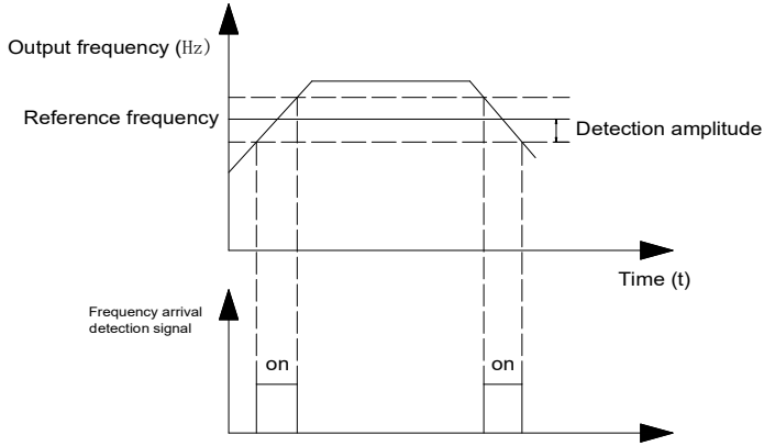
Figür 6-16 Frekansa ulaşma algılama diagramı
