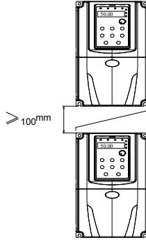
Tek Cihaz Montaj Diagramı
