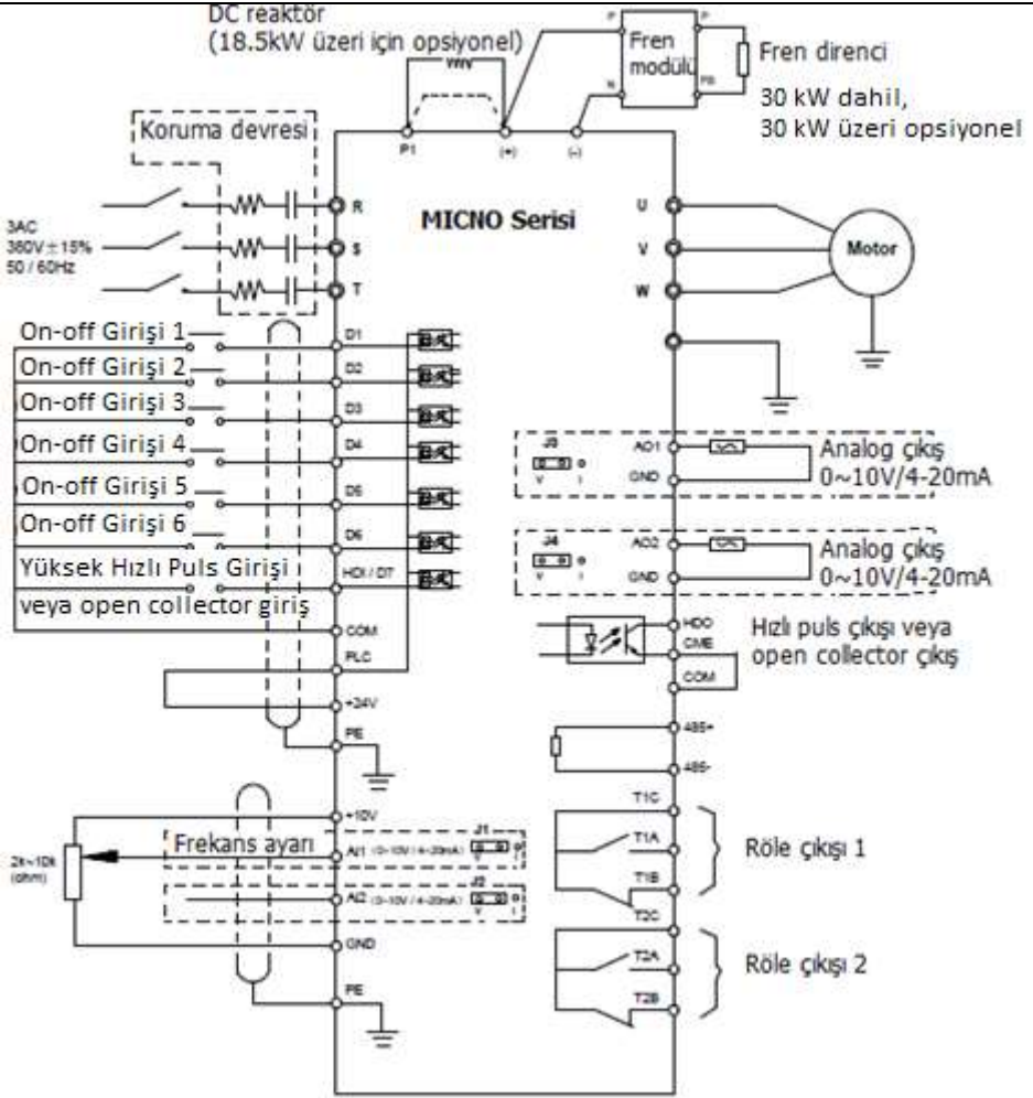
Figür 3-4 Bağlantı Diagramı (2,2 kW üzeri için geçerlidir)
