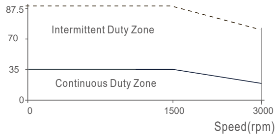
Torque(Nm)
