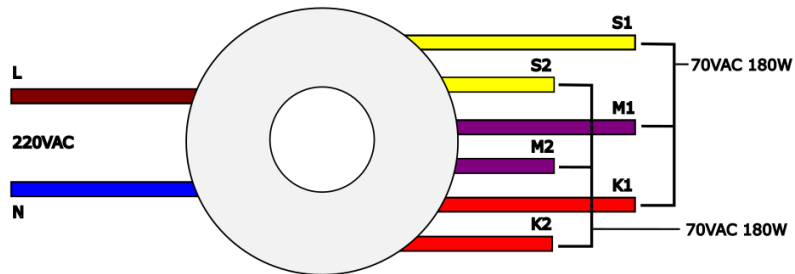
3 çıkışlı trafonun tek çıkışlı trafo gibi kullanılabilmesi için yapılması gereken bağlantı
