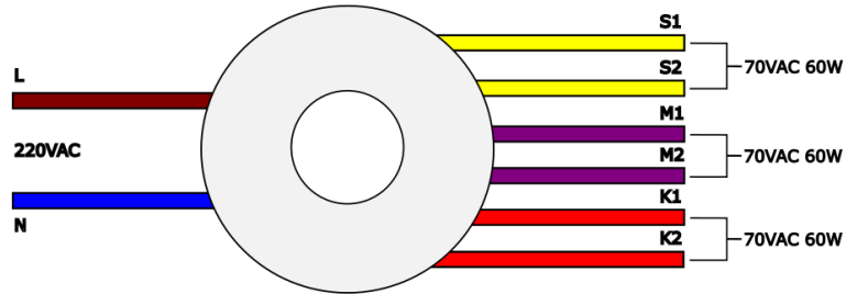
3 çıkışlı trafo bağlantısı
